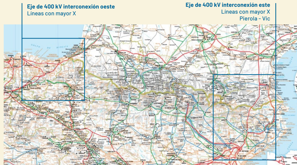
Figura 8. Líneas de los dos ejes principales de interconexión con Francia
