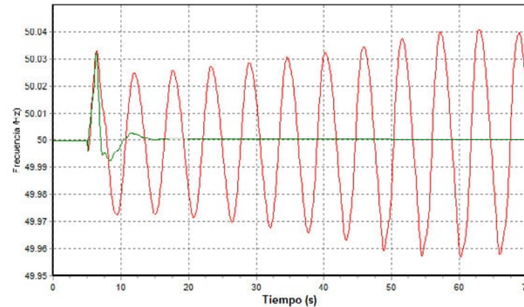
Figura 12. Respuesta dinámica del sistema teniendo en cuenta las necesidades estructurales del sistema para amortiguamiento de oscilaciones inter-área
